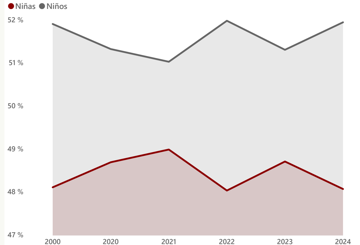
Nacimiento de niñas vs niños
